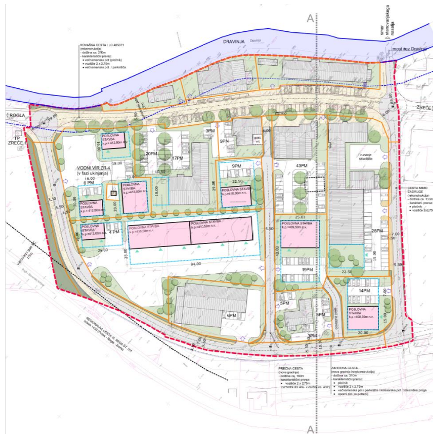
Slika 21: Predlog ureditvene situacije za območje poslovne zazidave Zgornje Zreče
