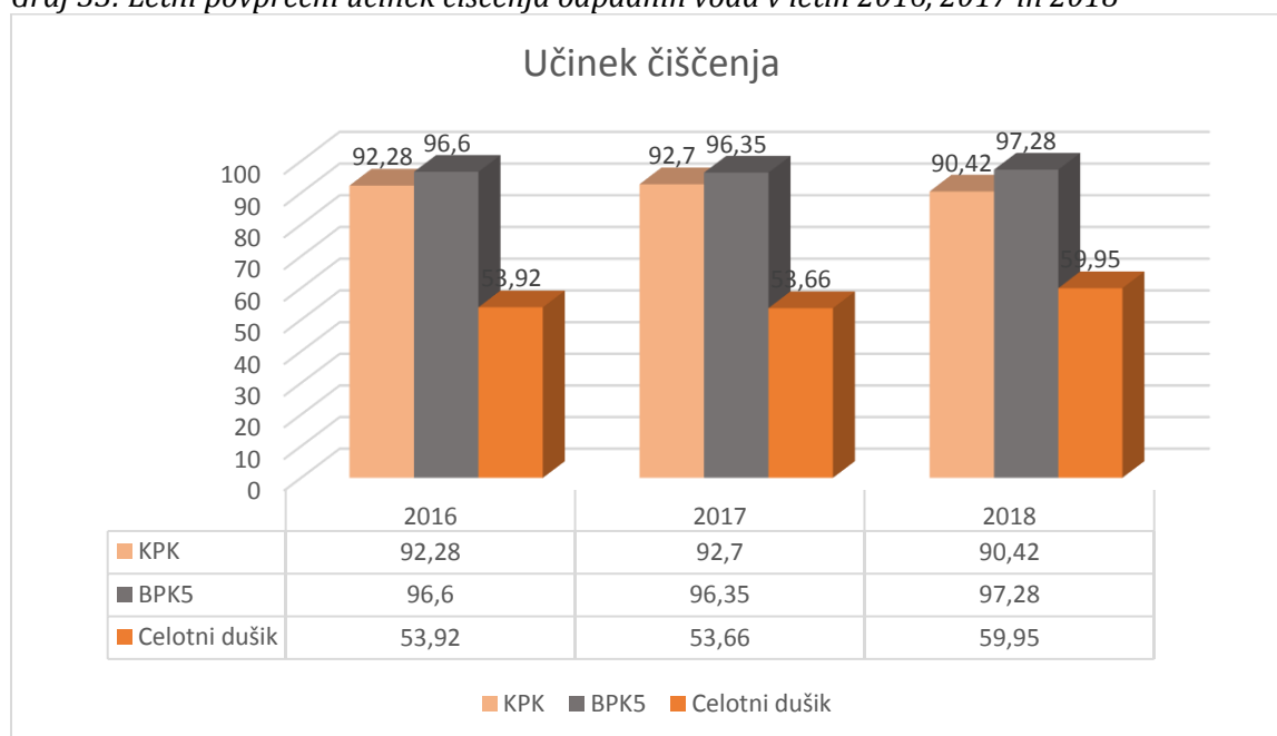
Graf 33: Letni povprečni učinek čiščenja odpadnih voda v letih 2016, 2017 in 2018
